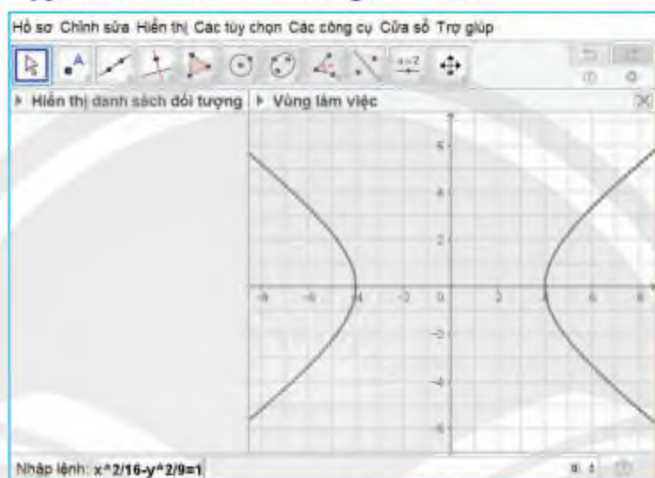
Hình 5. Vẽ hypebol theo phương trình chính tắc
