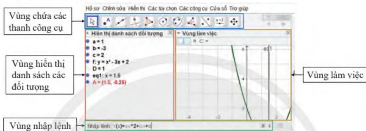
Hình 1. Các vùng làm việc của GeoGebra Classic 5
