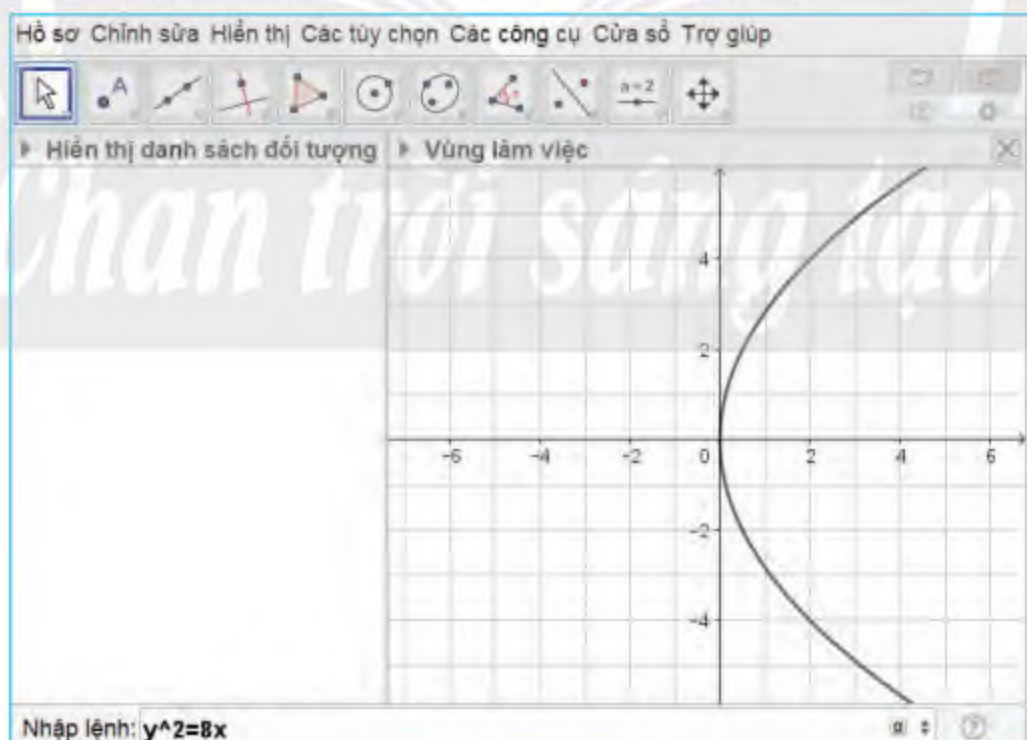
Hình 8. Vẽ parabol theo phương trình chính tắc
