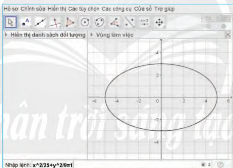
Hình 1. Vẽ elip theo phương trình chính tắc
